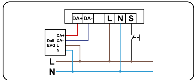
Master-Master-Anschluss mit Taster Master-Master connection + switch
